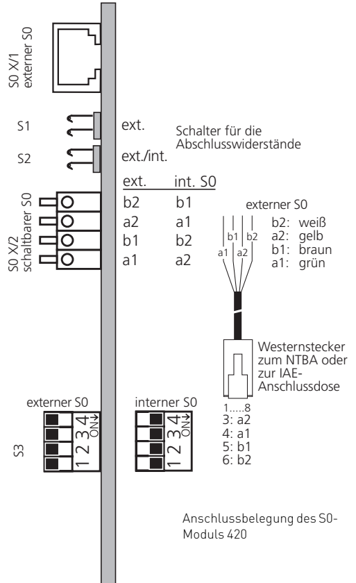
S0-Modul 420
