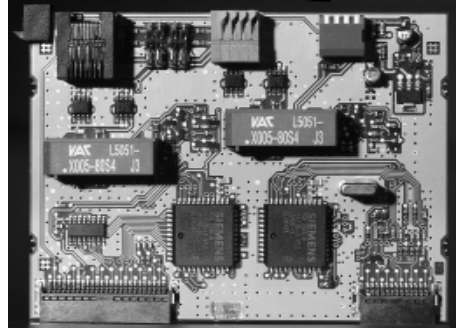
S0-Modul 420
